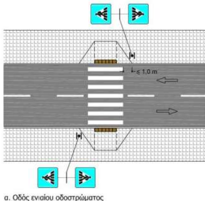
Εικόνα 6.8: Χωροθέτηση πινακίδων κατακόρυφης σήμανσης (Πηγή: ΟΜΟΕ, Τεύχος 10, Μέρος 1: Ισόπεδοι Κόμβοι, Αναθεωρημένη έκδοση: 03-09-2012)
