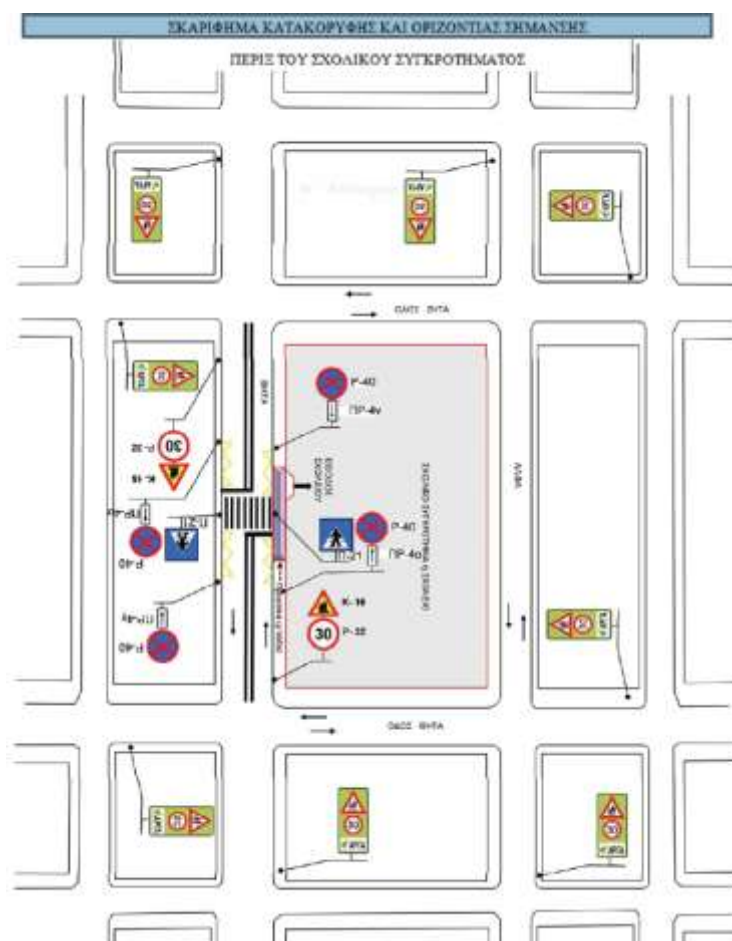
Εικόνα 6.9: Σκαρίφημα Κατακόρυφης & Οριζόντιας Σήμανσης πέριξ σχολικού συγκροτήματος
