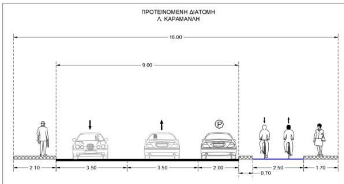
Εικόνα 6.14: Ενδεικτική Τυπική Διατομή Λ. Καραμανλή
