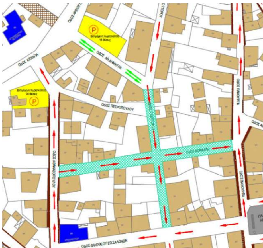
Εικόνα 3.6: Απόσπασμα από το σχέδιο που απεικονίζει την προτεινόμενη θέση της λαϊκής αγοράς (οδοί Κόκκαλη και Κοττορού)
