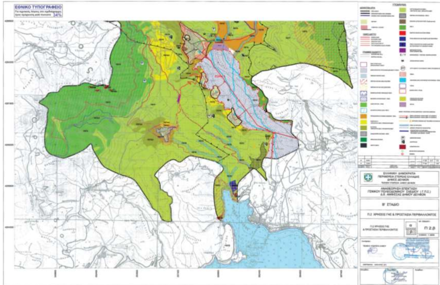
Εικόνα 2.5: «Χρήσεις γης & Προστασία περιβάλλοντος» - Χάρτης Π2.β του Γ.Π.Σ. Δ.Ε. Αμφισσας (ΦΕΚ 87/ΑΑΠ/2014)
