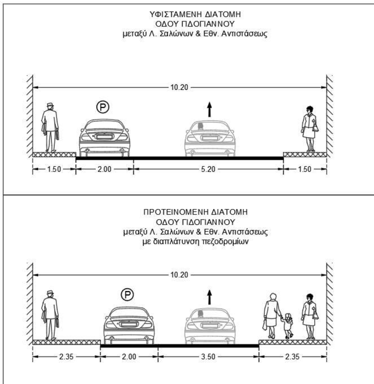
Εικόνα 6.12: Ενδεικτική Τυπική Διατομή οδού Γιδογιάννου, μεταξύ Λ. Σαλώνων & Εθν. Αντίστασης, με διαπλάτυνση πεζοδρομίων
