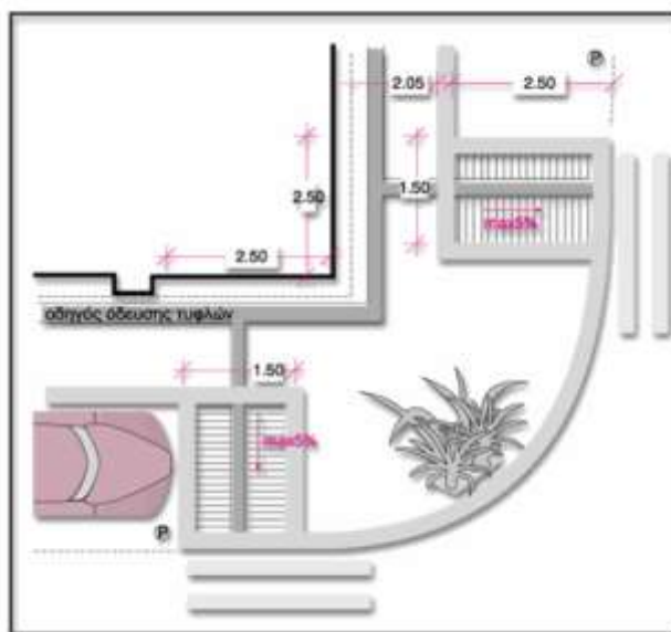
Εικόνα 6.7: Ενδεικτική διαμόρφωση εγκιβωτισμού θέσεων στάθμευσης
