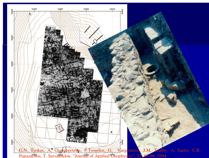
Εικ. 5. Χαρτογραφημένος κάνναβος, μετρήσεις και επεξεργασία τους, παραγωγή χάρτου θαμμένων δομών και ένα αποτέλεσμα προσανατολισμένης ανασκαφικής έρευνας.
