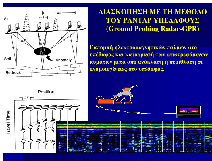
Εικ. 1. Σχηματικό διάγραμμα μετρήσεων με γεωραντάρ.
