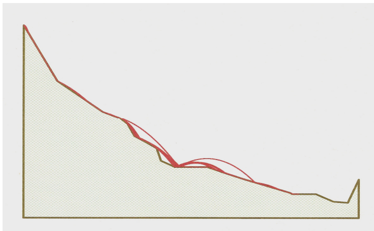
Εικ. 3. Τυπική ανάλυση τροχιάς βραχοπτώσεων σε δύο διαστάσεις (λογισμικό rockfall, Εργαστήριο Δομικής Μηχανικής & ΣΤΕ, ΕΜΠ).
