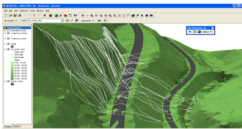
Εικ. 4. Τυπική ανάλυση τροχιάς βραχοπτώσεων σε τρεις διαστάσεις (λογισμικό rockfall analysis 3-D, Εργαστήριο Δομικής Μηχανικής & ΣΤΕ, ΕΜΠ).
