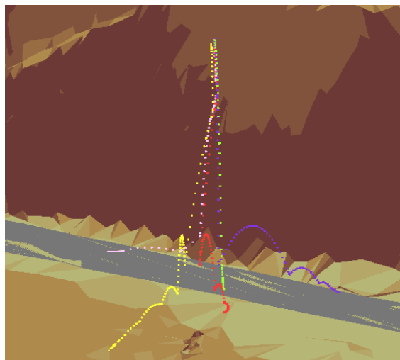
Εικ. 5. Ανάδειξη του φαινομένου της εγκάρσιας διασποράς των τροχιών λόγω αναγλύφου με ανάλυση σε τρεις διαστάσεις (λογισμικό rockfall analysis 3-D, Εργαστήριο Δομικής Μηχανικής & ΣΤΕ, ΕΜΠ).
