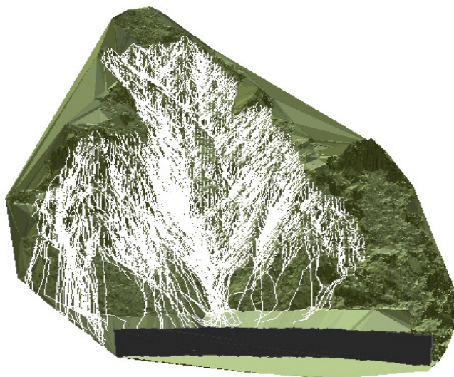
Εικ. 7. Σχεδιασμός φράχτη ανάσχεσης βραχοπτώσεων με ανάλυση σε τρεις διαστάσεις, στοχαστική ανάλυση. Ψηφιοποίηση του εδάφους με Laser Scanner (λογισμικό rockfall analysis 3-D, Εργαστήριο Δομικής Μηχανικής & ΣΤΕ, ΕΜΠ).
