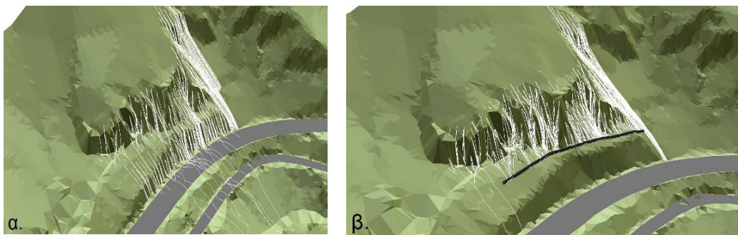
Εικ. 6. Σχεδιασμός μέτρων προστασίας με ανάλυση σε τρεις διαστάσεις, (α) χωρίς φράχτη, (β) με φράχτη (λογισμικό rockfall analysis 3-D, Εργαστήριο Δομικής Μηχανικής & ΣΤΕ, ΕΜΠ).
