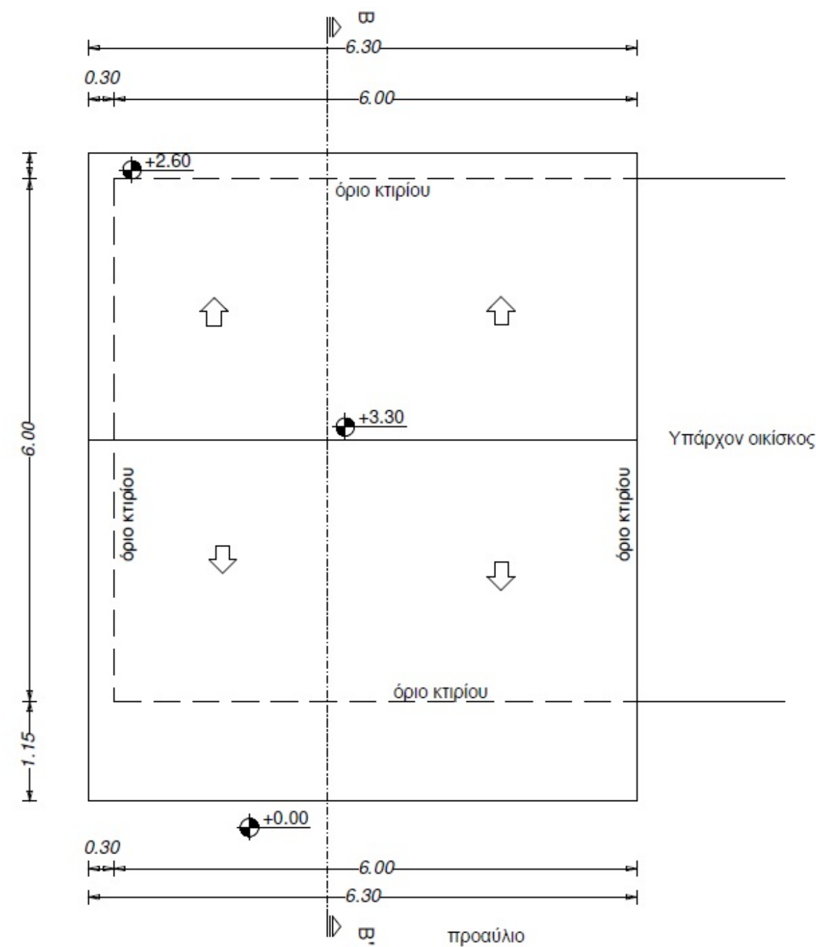
ΚΑΤΟΨΗ ΣΤΕΓΗΣ κλίμακα 1:50
