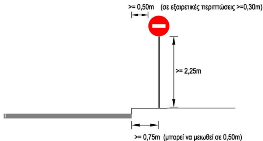
Εικόνα 5.1: Τοποθέτηση Πινακίδας σε Αστική Οδό με Πεζοδρόμιο (ταχύτητα \leq 50\text{km/h} )
