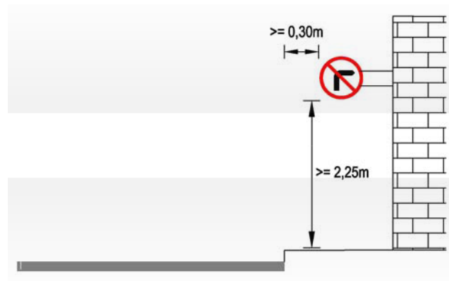
Εικόνα 5.2: Στήριξη Πινακίδας σε Τοίχο σε Αστικές Περιοχές
