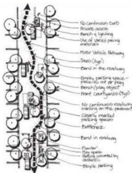
Εικόνα 4.7. Πρότυπο σχεδιασμού δρόμου ήπιας κυκλοφορίας τύπου «woonerf»
