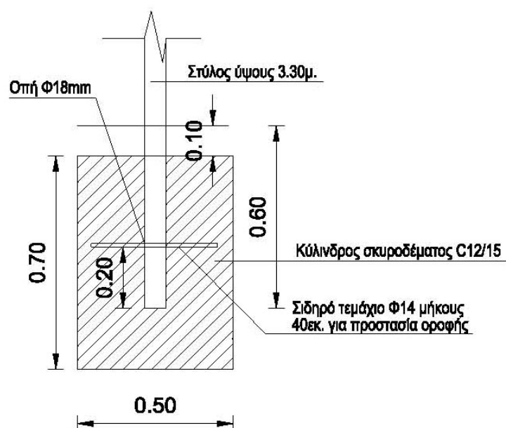
Εικόνα 5.4: Θεμελίωση Στόλων Στήριξης Πινακίδων
